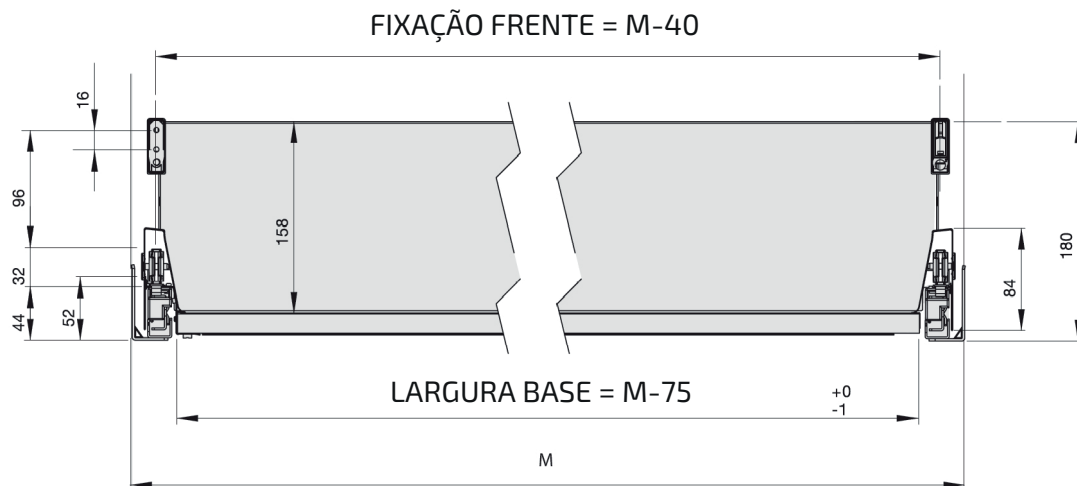
Gaveta H116 com tubo lateral - traseira de gaveta alta
