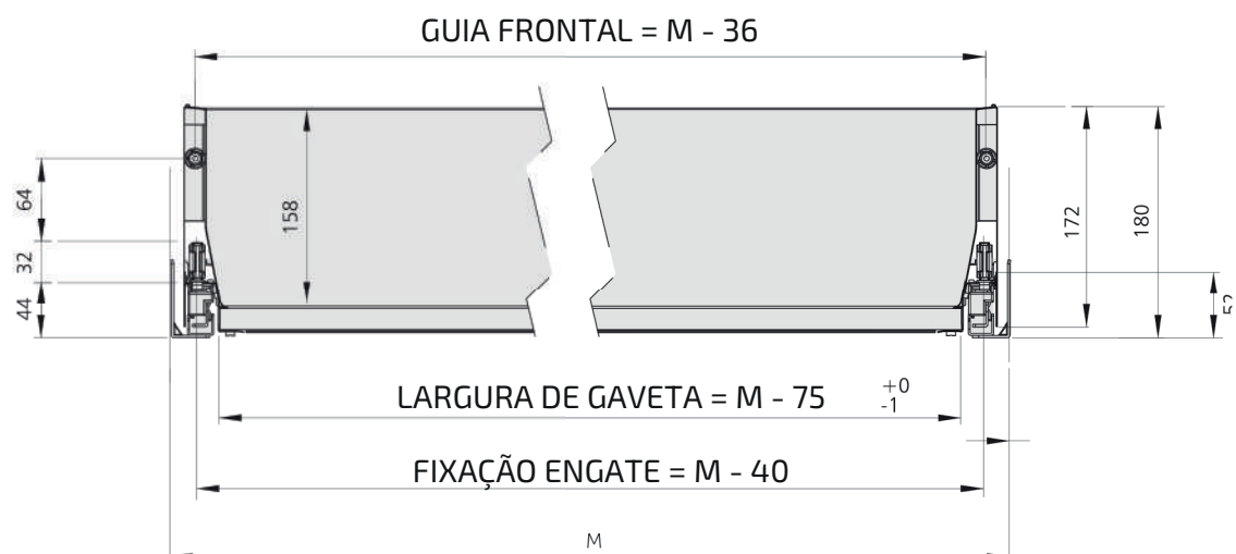
Gaveta H172 com traseira MDF para gaveta alta
